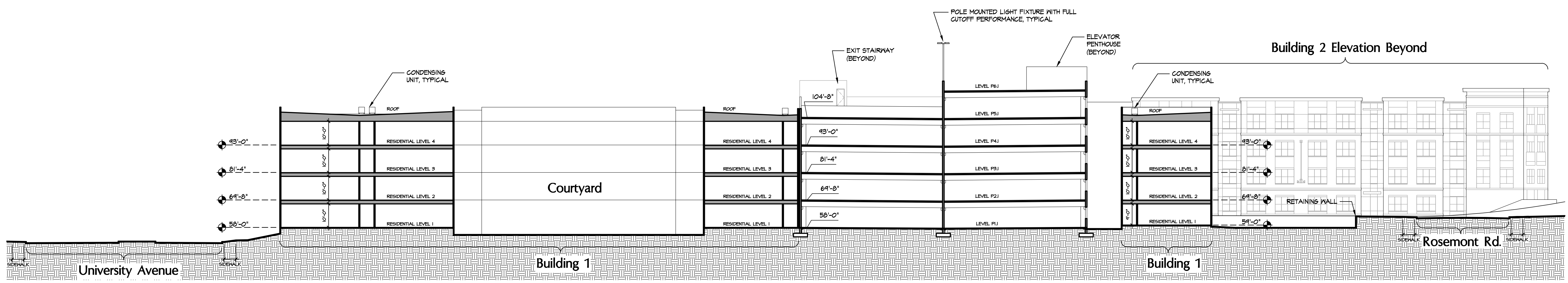
2 Site Section SCALE: 1" = 20'-0"
