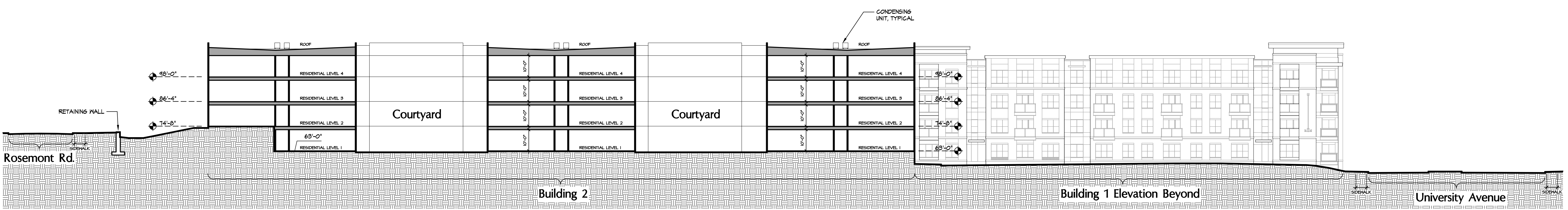
1 Site Section SCALE: 1" = 20'-0"
