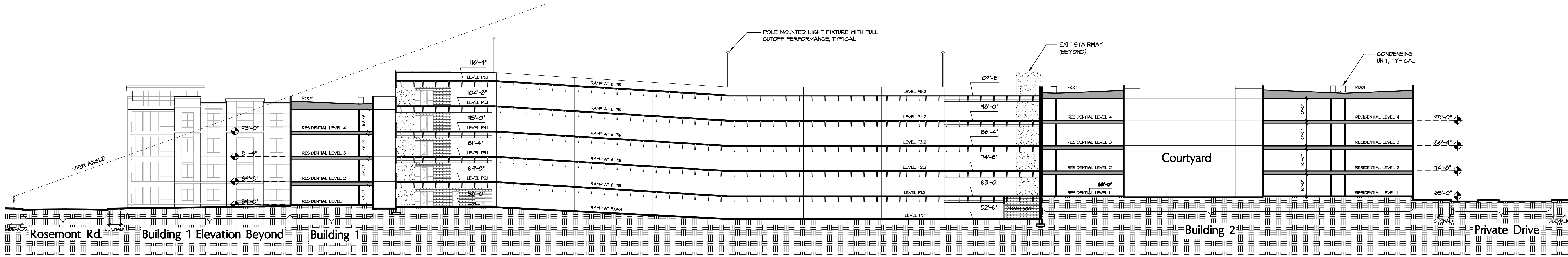
3 Site Section SCALE: 1" = 20'-0"
